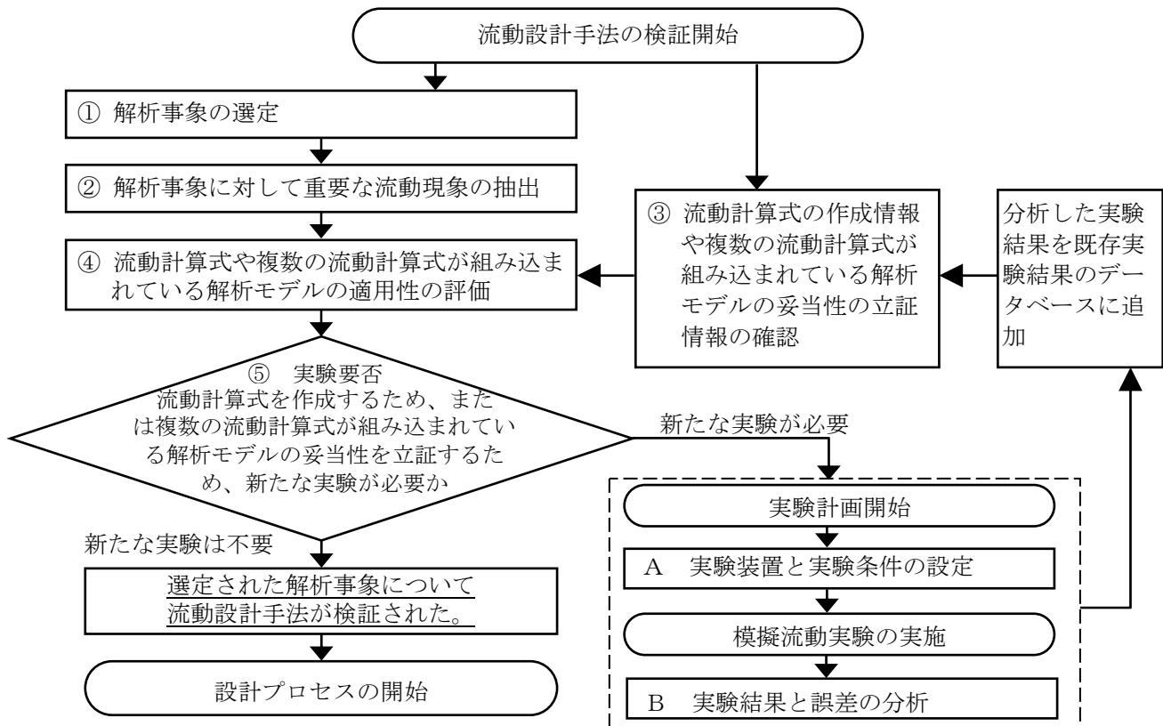
図-1 最新の妥当性立証手法に基づくFBR流動設計手法の検証方法の手順
