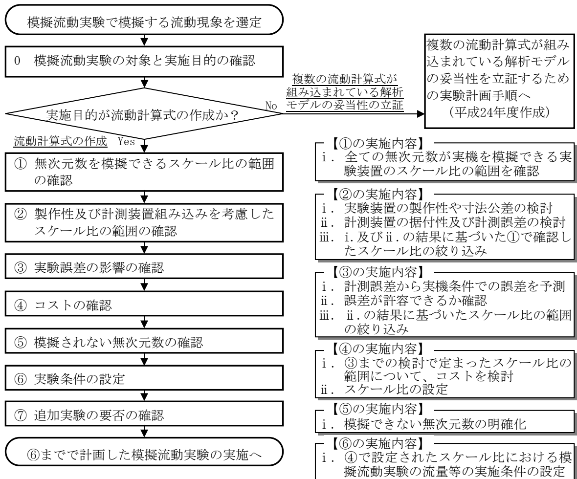
図-2 流動計算式を作成するための模擬流動実験の実験計画手順
